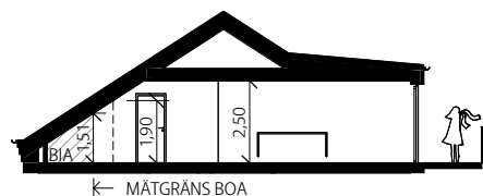
TYPSEKTION 1, VIND
