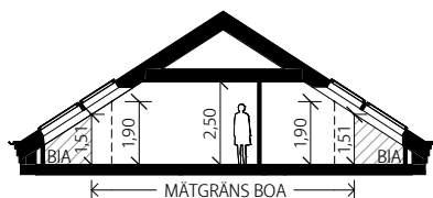
TYPSEKTION 2, VIND
