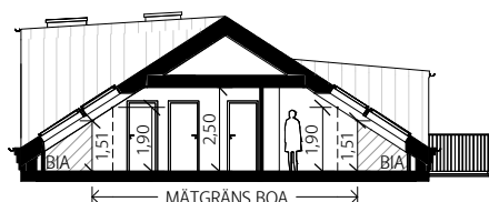
TYPSEKTION 2, VIND
