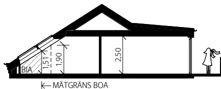
TYPSEKTION 1, VIND
